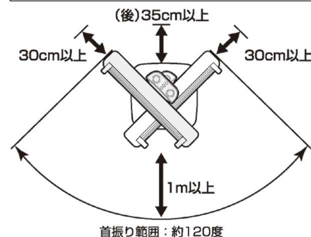
ヒーターユニットが横向きの場合(上から見た図)
